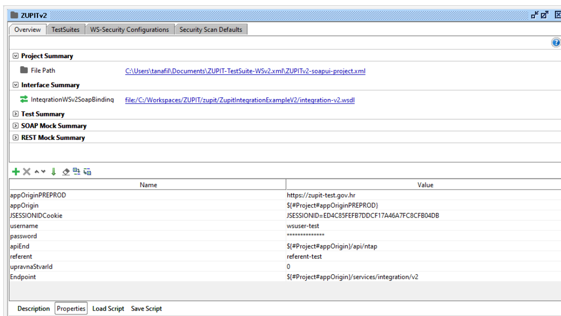
Slika 3. Primjer konfiguracija SoapUI projekta za spajanje na testni server
