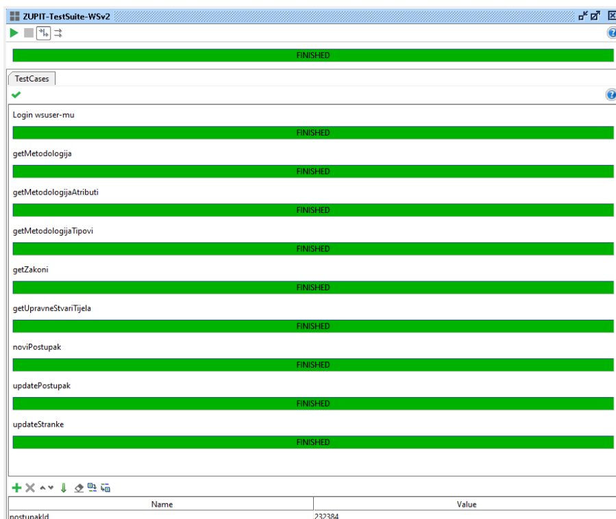
Slika 5. Primjer uspješno pokrenutog TestSuite-WSv2 primjera
