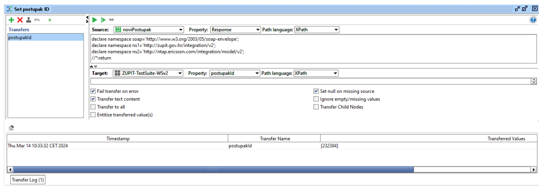
Slika 7. Primjer uspješno postavljenog parametra postupakId
